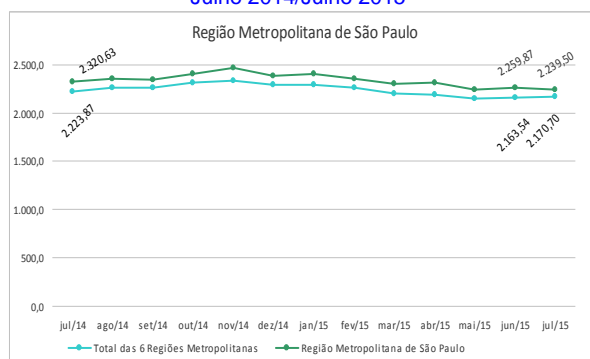
Rendimento médio real habitual dos ocupados Total das 6 Regiões Metropolitanas e RM de São Paulo Julho 2014/Julho 2015
